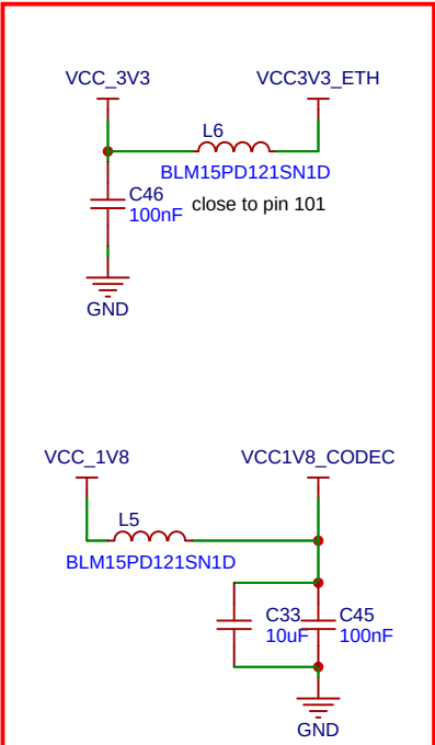
滤波
